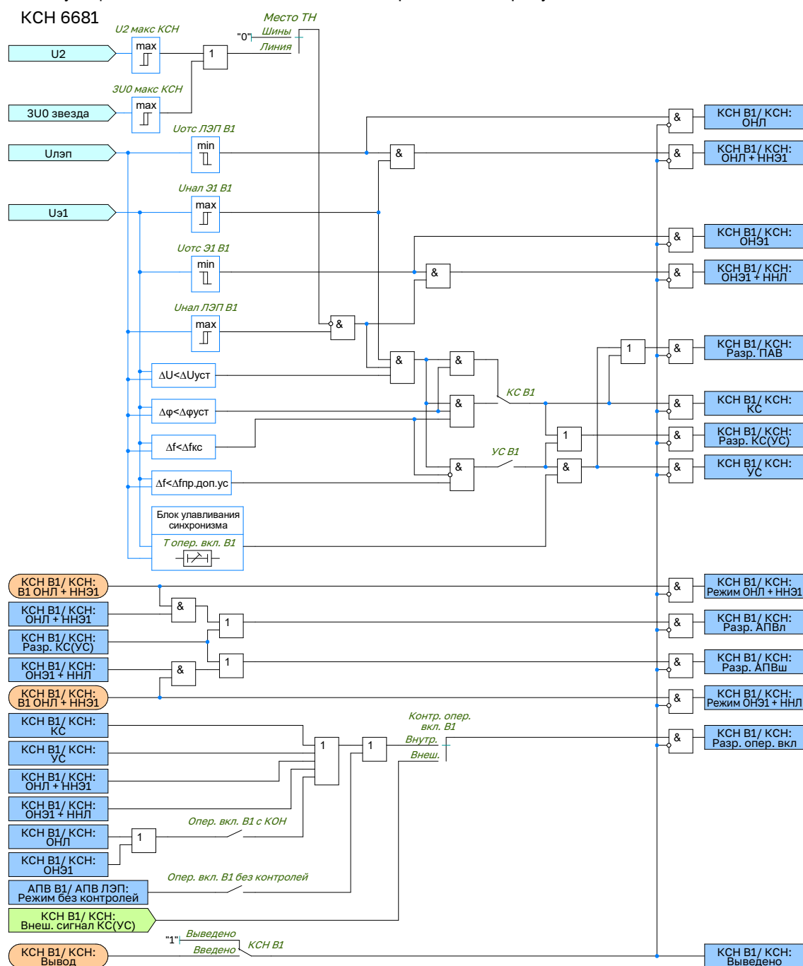
Рисунок 2.66 – Функциональная схема логики КСН В1
