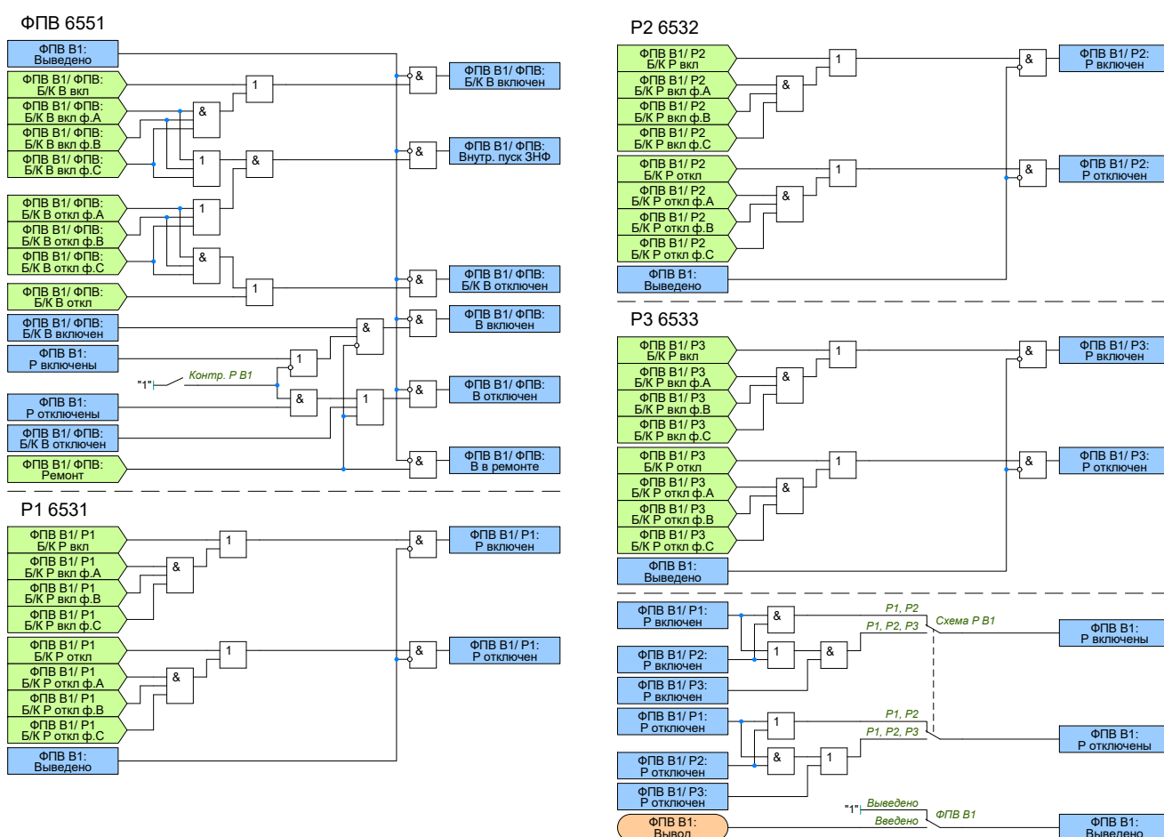
Рисунок 2.81 – Функциональная схема логики ФПВ В1
