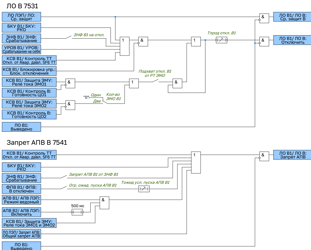
Рисунок 2.79 – Функциональная схема логики отключения В1 и запрета АПВ В1
