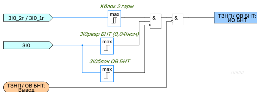
Рисунок 2.43 – Функциональная схема логики органа выявления БНТ
