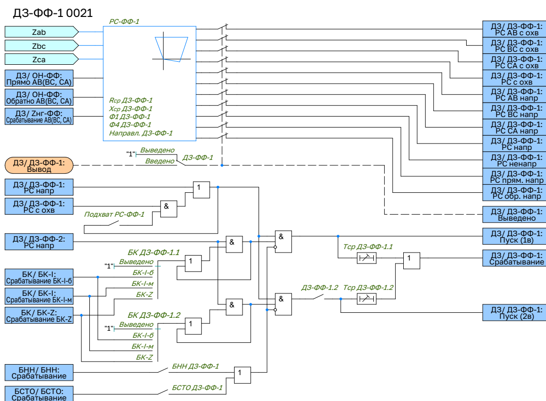
Рисунок 2.31 – Функциональная схема логики ДЗ-ФФ-1
