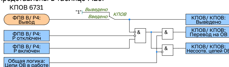
Рисунок 2.87 – Функциональная схема логики контроля перевода на ОВ
