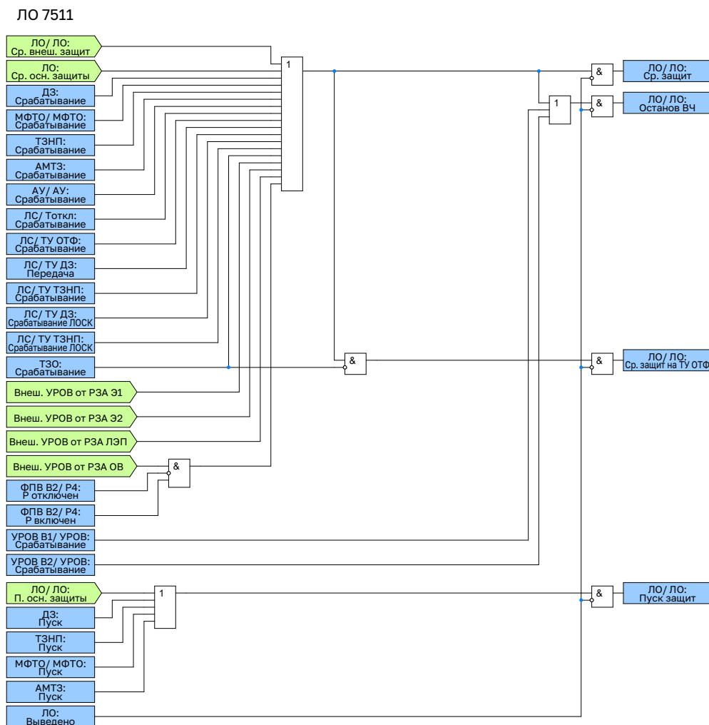
Рисунок 2.77 – Функциональная схема общей логики отключения
