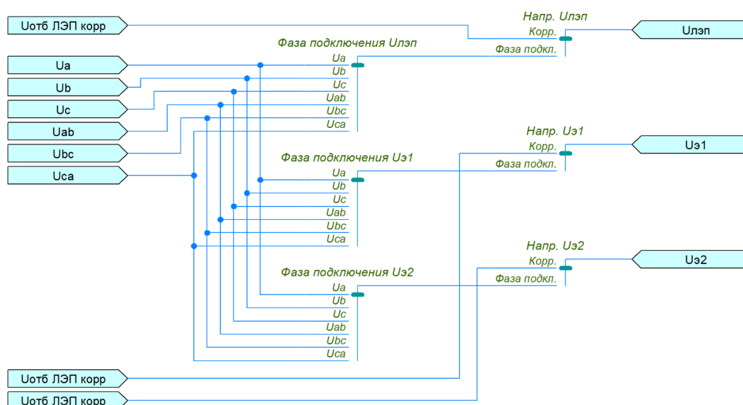
Рисунок 2.88 – Функциональная схема настройки аналоговых значений U_{лэп} , U_{э1} , U_{э2}
