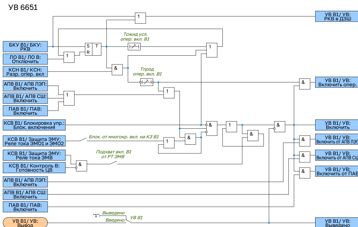
Рисунок 2.80 – Функциональная схема управления выключателем В1
