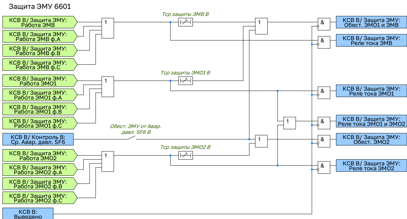
Рисунок 2.74 – Функциональная схема логики защиты ЭМУ выключателя
