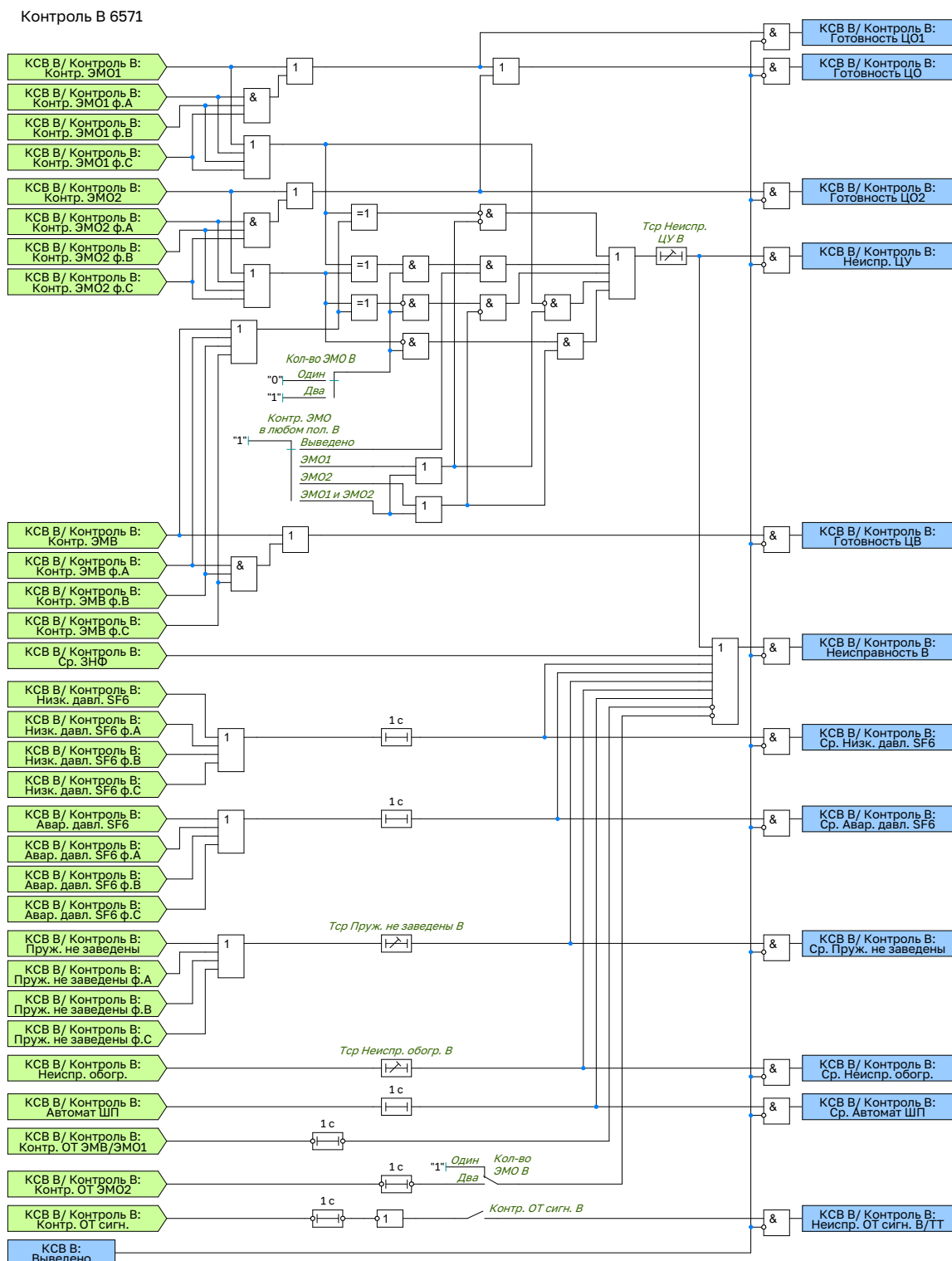
Рисунок 2.72 – Функциональная схема логики контроля выключателя
