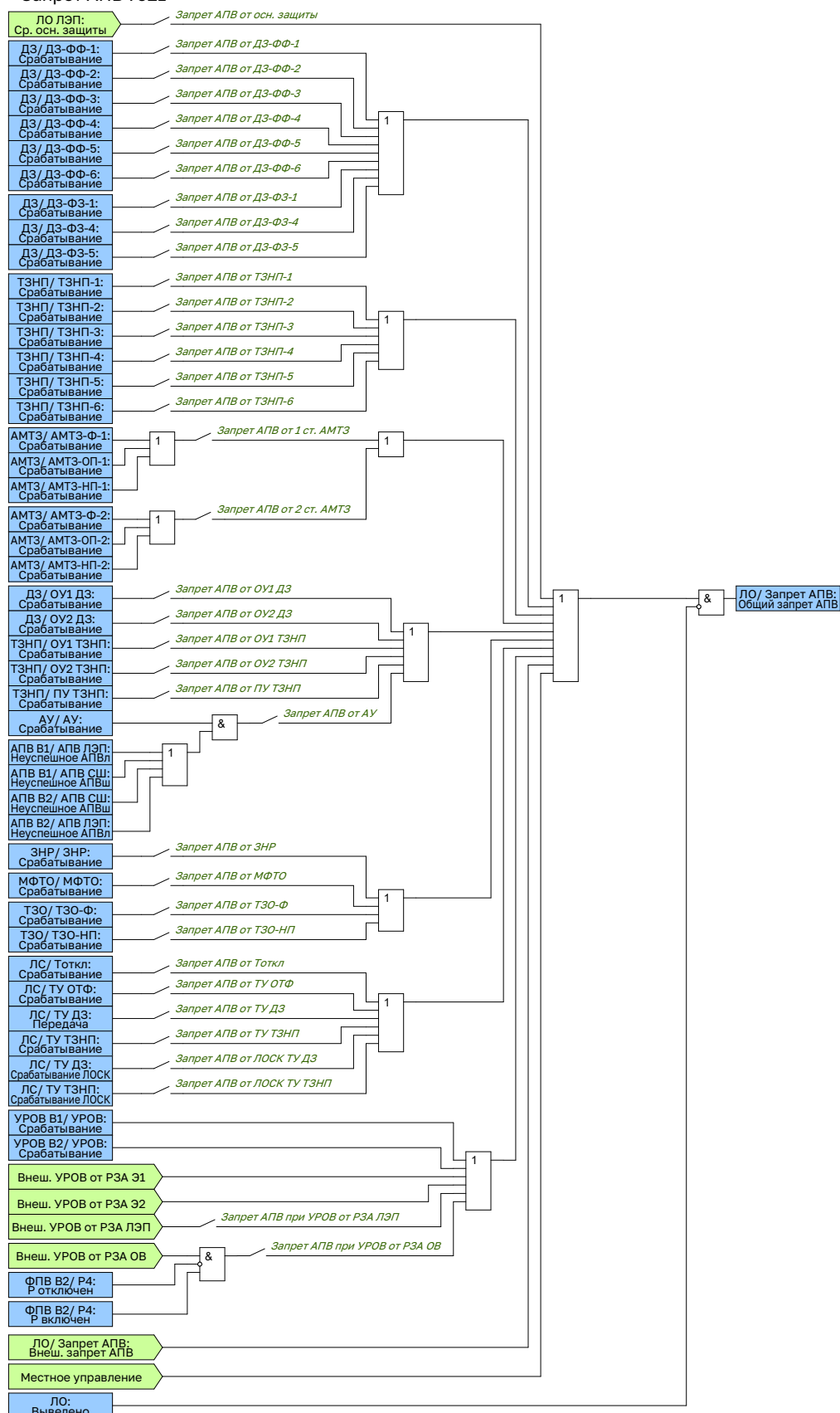
Рисунок 2.78 – Функциональная схема общей логики запрета АПВ
