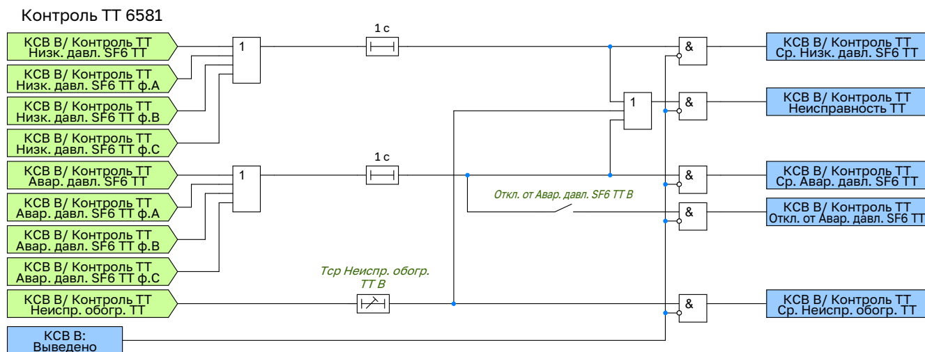
Рисунок 2.73 – Функциональная схема логики контроля ТТ выключателя
