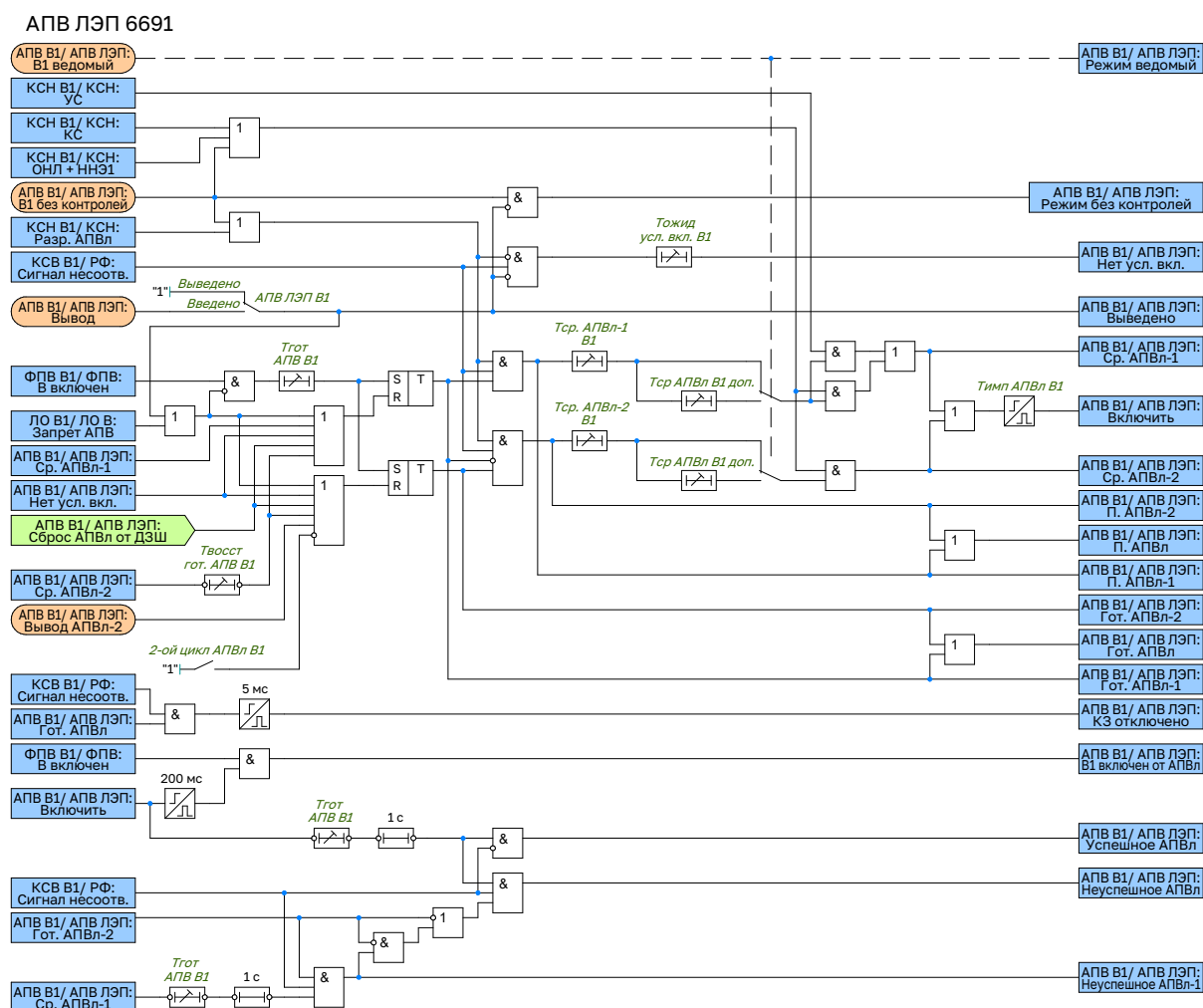
Рисунок 2.67 – Функциональная схема логики АПВ В1 ЛЭП
