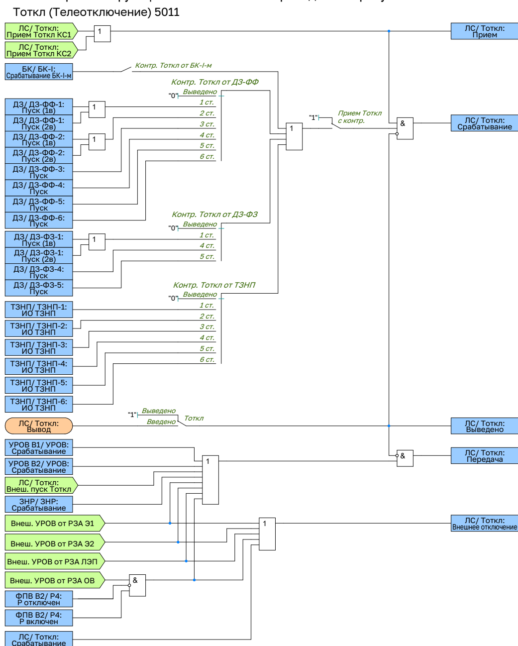
Рисунок 2.59 – Функциональная схема логики телеотключения
